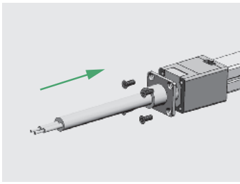
Fest braketten på PC-skallet med 4 stk skruer, på PC-skallet.
